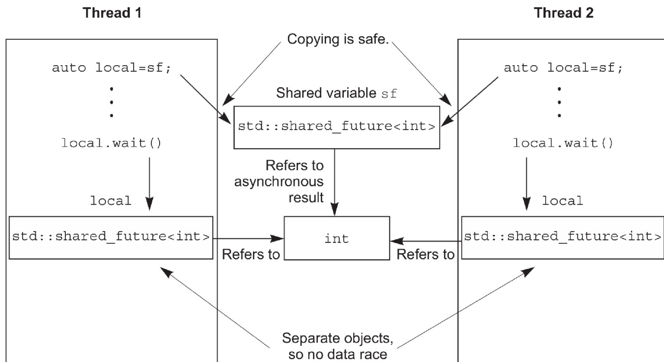
图4.1 使用多个 std::shared_future 对象来避免数据竞争
