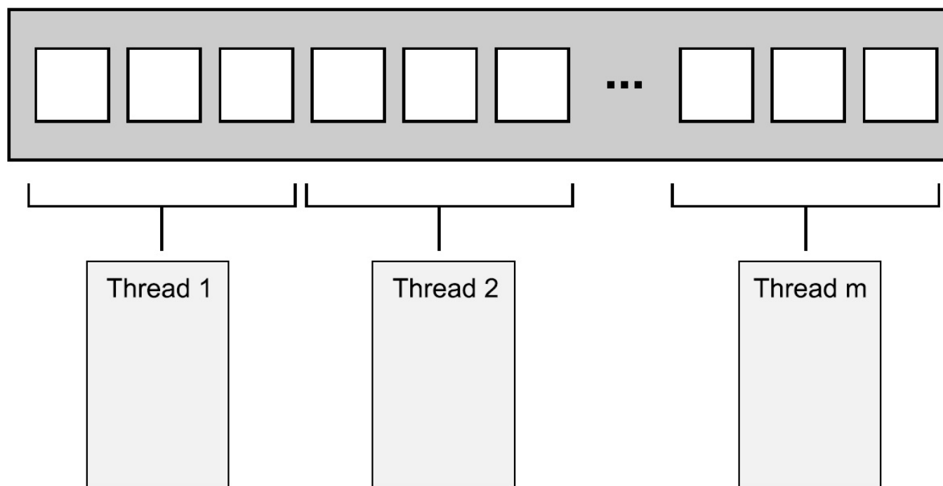
图8.1 向线程分发连续的数据块
