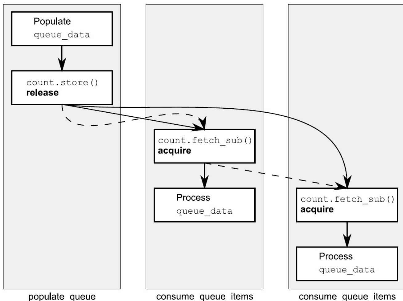
图5.7 清单5.11中对队列操作的释放顺序
