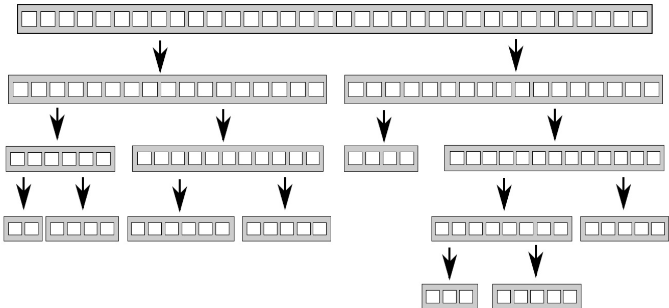
图 8.2 递归划分数据
