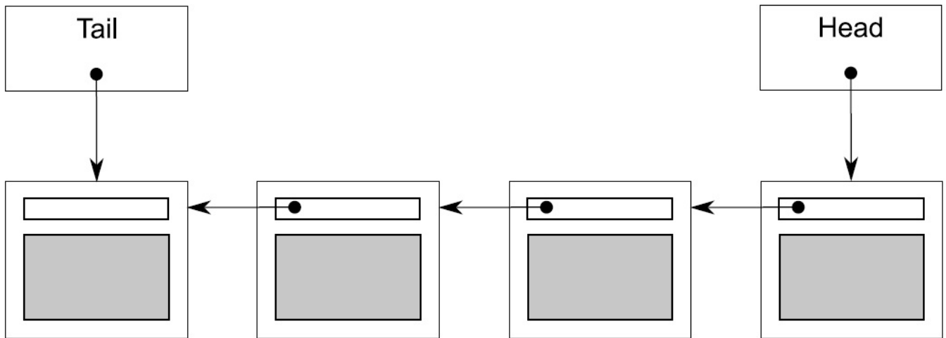
图6.1 用单链表表示的队列
