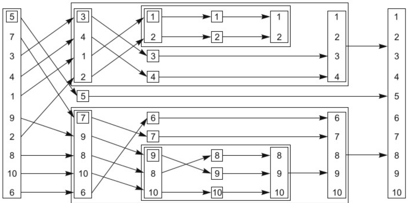
图4.2 FP-模式的递归排序
