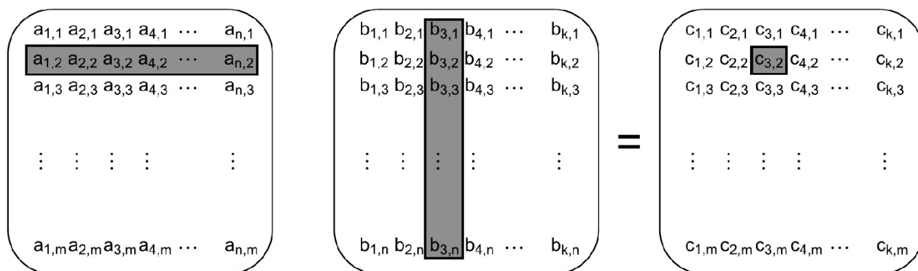
图8.3 矩阵相乘
